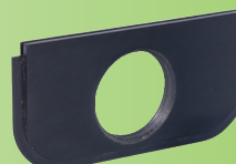
Un orificio roscado de 1" RPA para pata de montaje en tubería o glándula de cable de 1".
